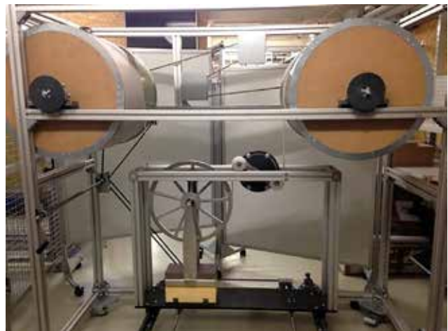
Kabelprüfstand in der Erprobung
