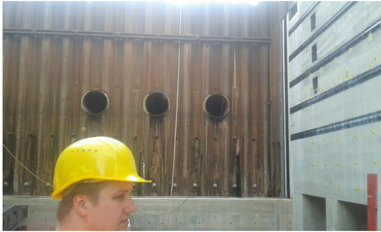
Hochwassersicherung mit Öffnungen zum gezielten Fluten der Baugrube bei Überschreitung des 20- jährigen Bauhochwassers
